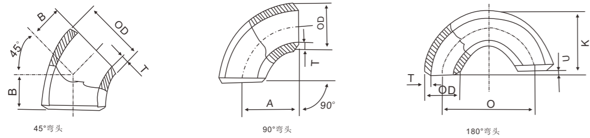
单位:毫米
