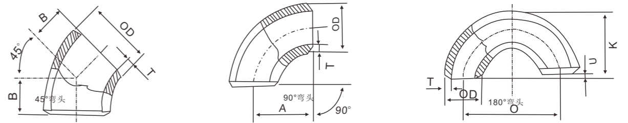
单位:毫米
